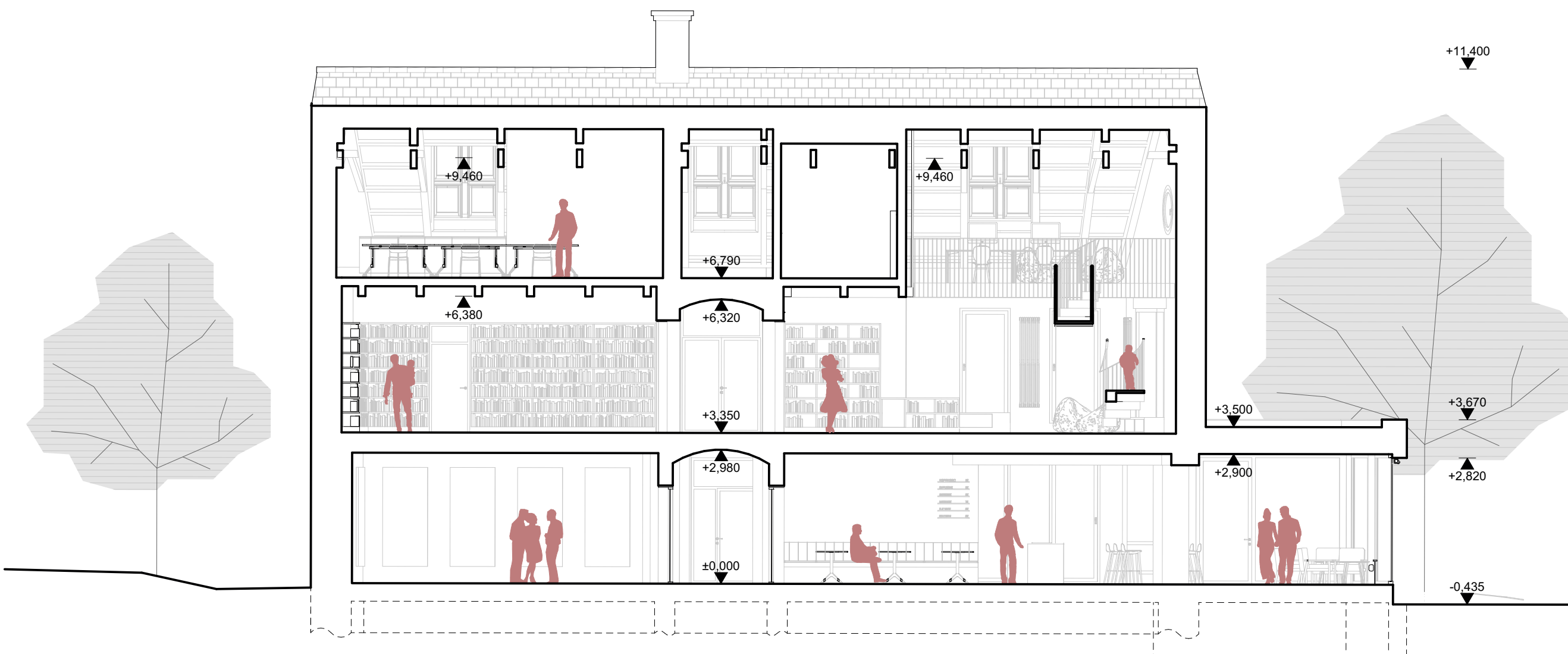
ŘEZ D-D'
